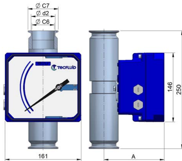
Sanitary connection CLAMP ISO 2852 (EN 1.4404)
