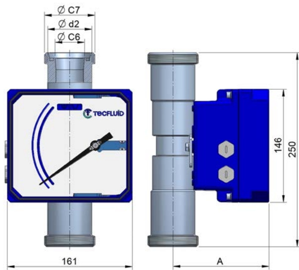
Sanitary connection DIN 11851 (EN 1.4404)
