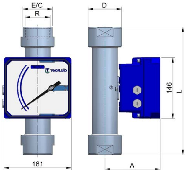
Threaded connection BSP / NPT (EN 1.4404)
